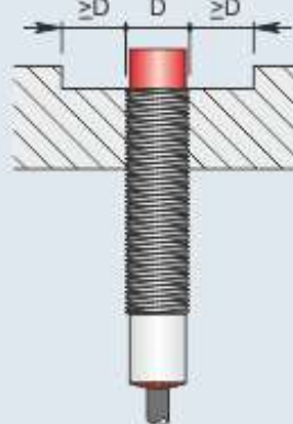
Montaggio sporgente
